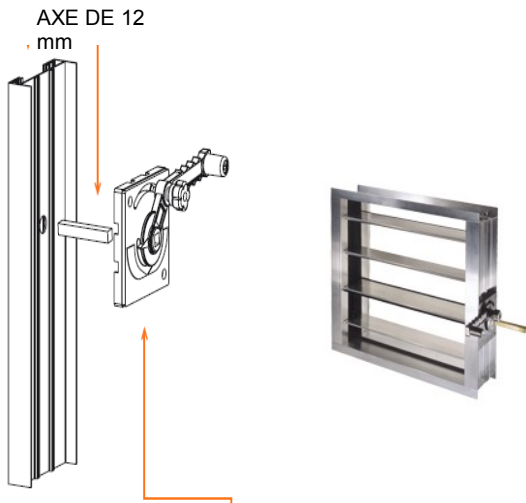
Commande manuelle Avec secteur de blocage
